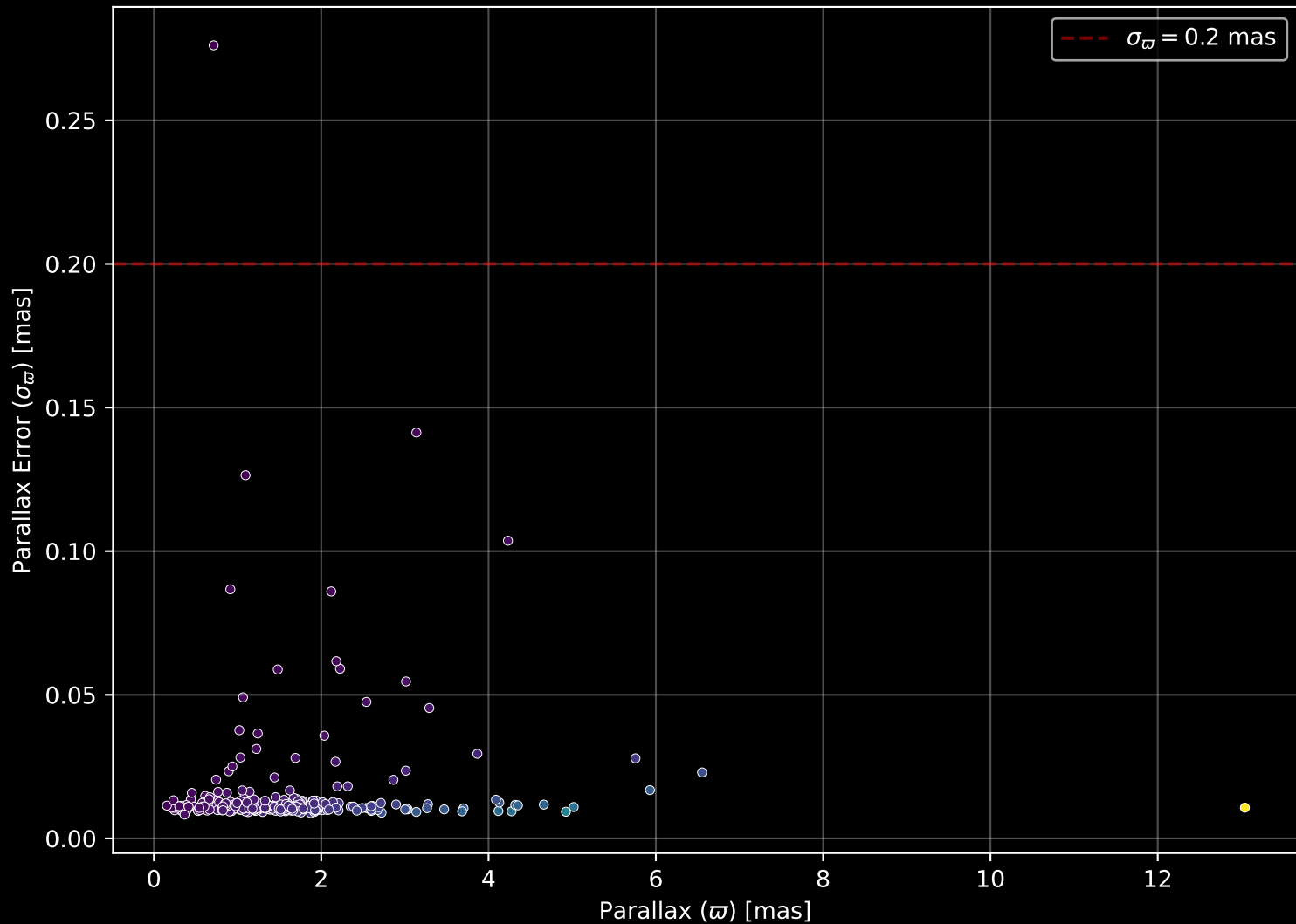
GALAH DR4 Field: [1179] Parallax Quality (n= 295)
