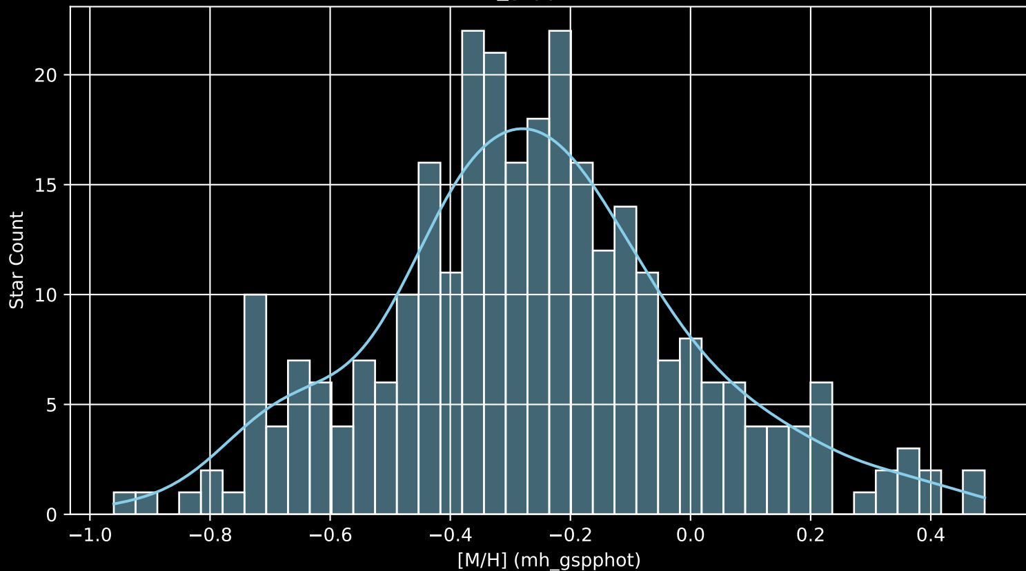
GALAH DR4 Field: [1179] [M/H] (mh_gspphot) (n= 294)
