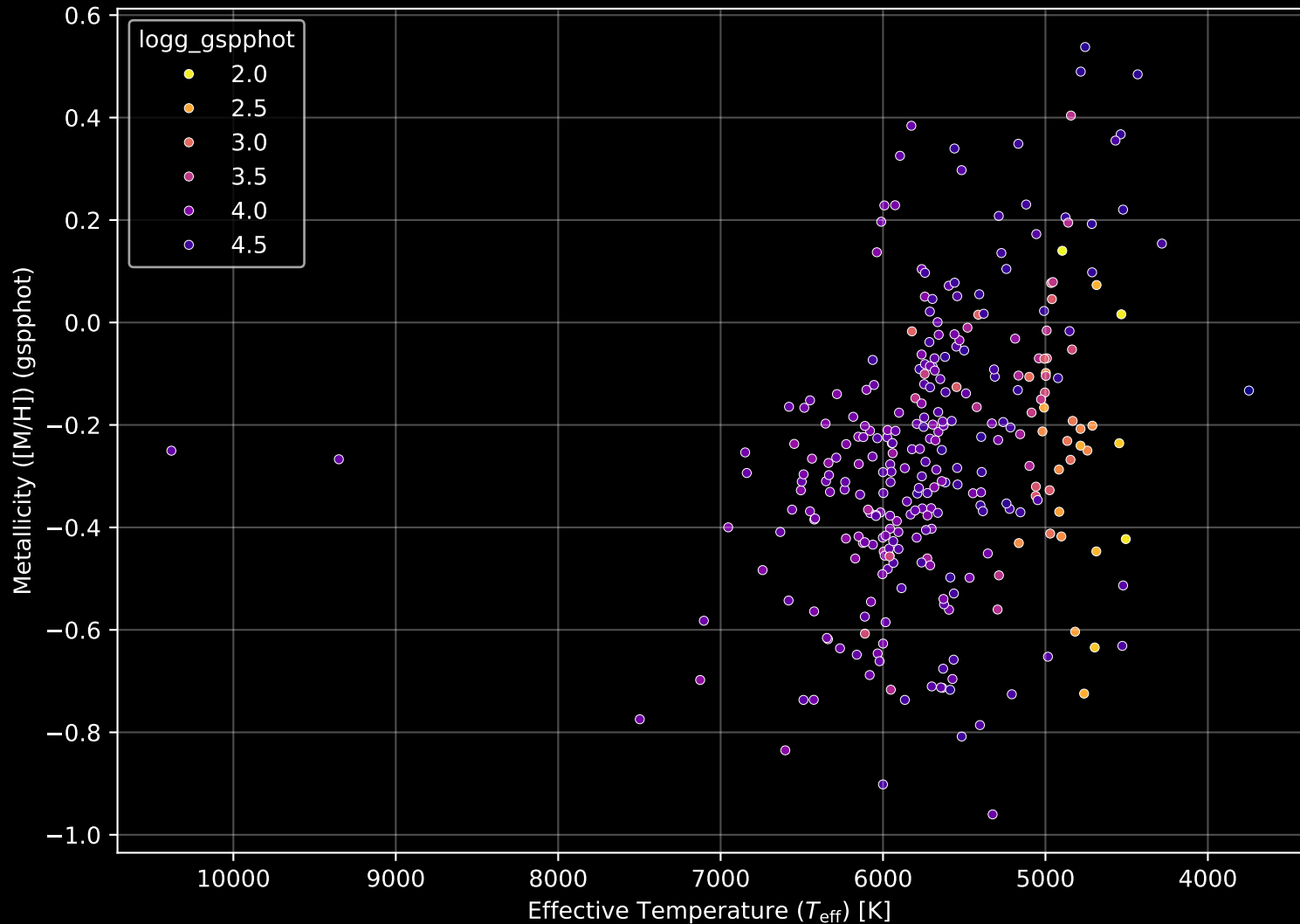
GALAH DR4 Field: [1179] Stellar Population Parameters (n= 295)
